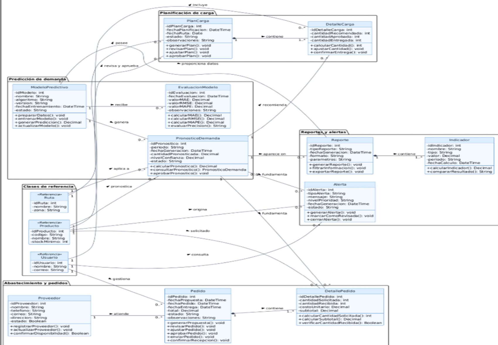
Diagrama de clases 2 Predicción, cargas, abastecimiento y reportes
